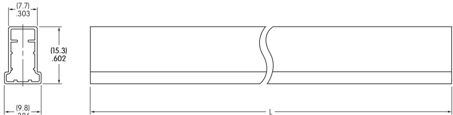
Stick-Tube Dimensions
